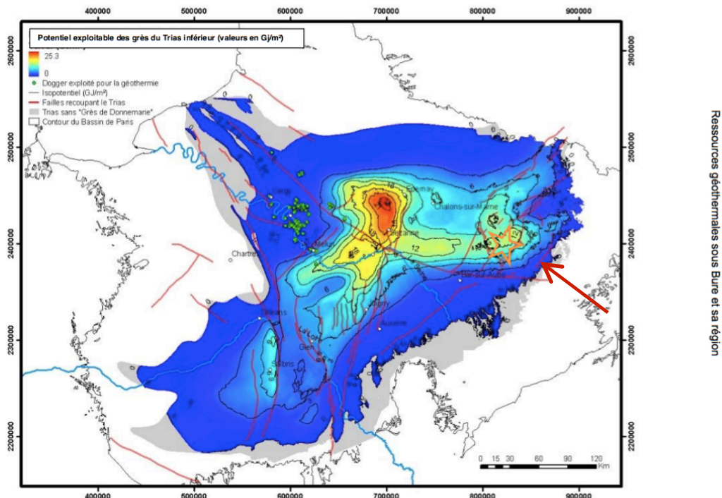
Figure 7 - Carte du potentiel géothermique, souligné par des isopotentiels à un pas de 3 GJ/m 3 des grès de Donnemarie situés dans la partie occidentale du Bassin parisien et des grès du Buntsandstein dans sa partie orientale (Lorraine), avec position du site de Bure (flèche orange) (modifié Bouchot et al., 2008).
